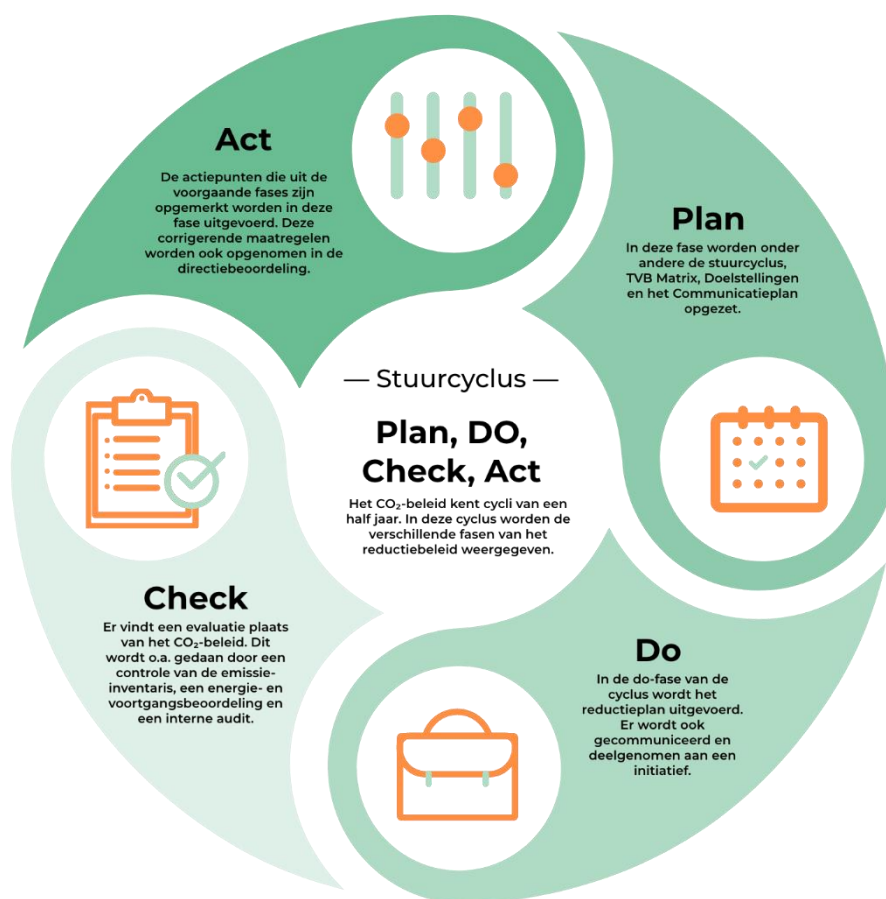
Figuur 1: PDCA-cyclus
